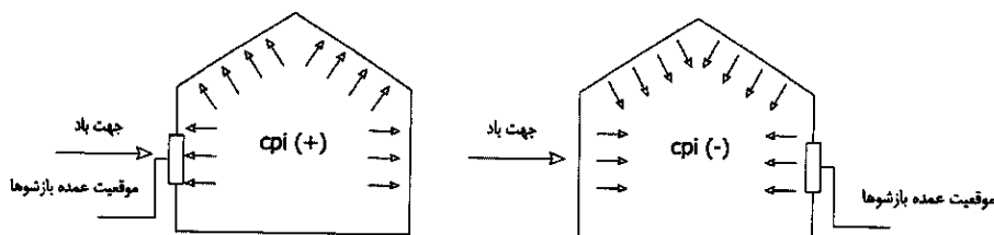
شکل ۶-۱۰-۱۲ ضریب اثر بازو C_{pi}
