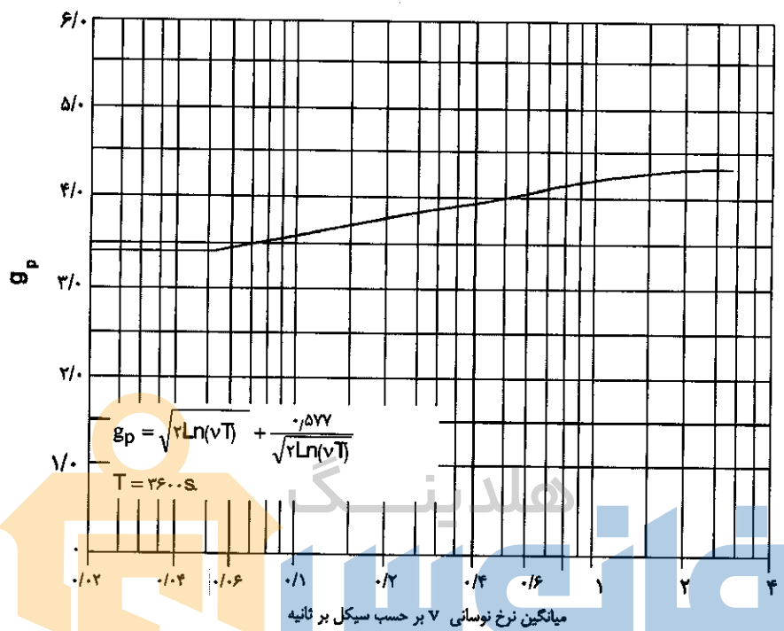
شکل پ-۶-۴ ضریب پیشینه آماری باز ( g_p )
