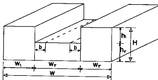
شکل ۱۱-۱۰-۶ نسبت ابعادی ساختمان‌های با بام پله‌ای تخت
