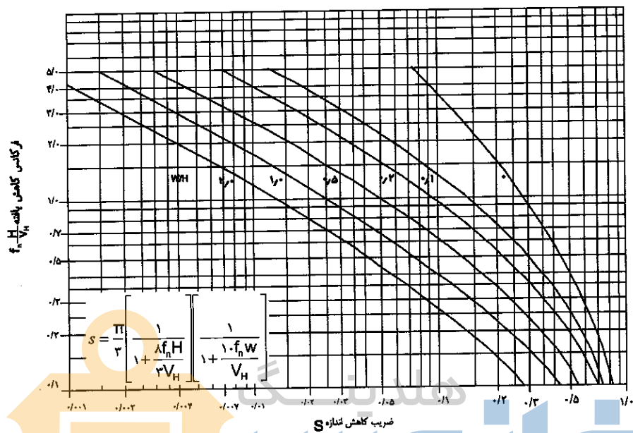
شکل پ-۶-۴-۲ ضریب کاهش اندازه (S)
