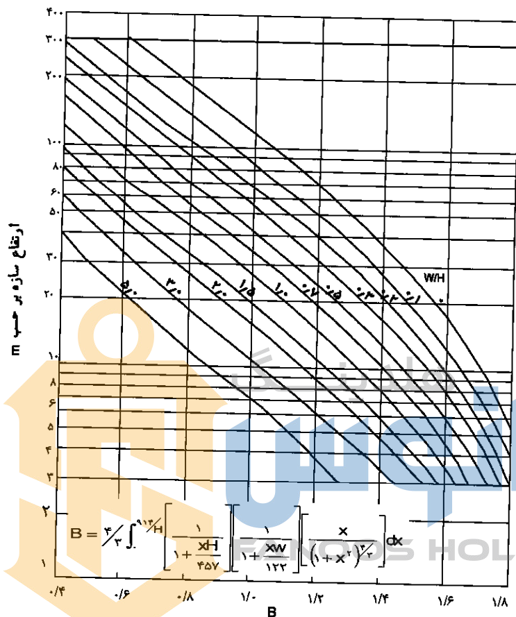
شکل پ-۶-۱ ضریب آشفته‌گی محیط ساختمان (B)
