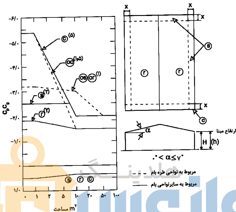
شکل ۶-۱۰-۶ ضرایب ترکیبی فشار و مکش خارجی C_p C_g برای طراحی پوشش‌ها و اجزاء بام (با زاویه شیب کمتر از ۷ درجه، یا یا بدون طره)
