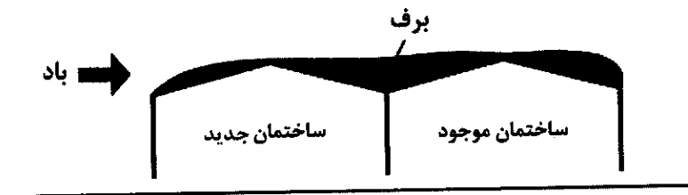
شکل ۷-۶-۱۱ اثر بار برف روی پام ساختمانهای موجود
