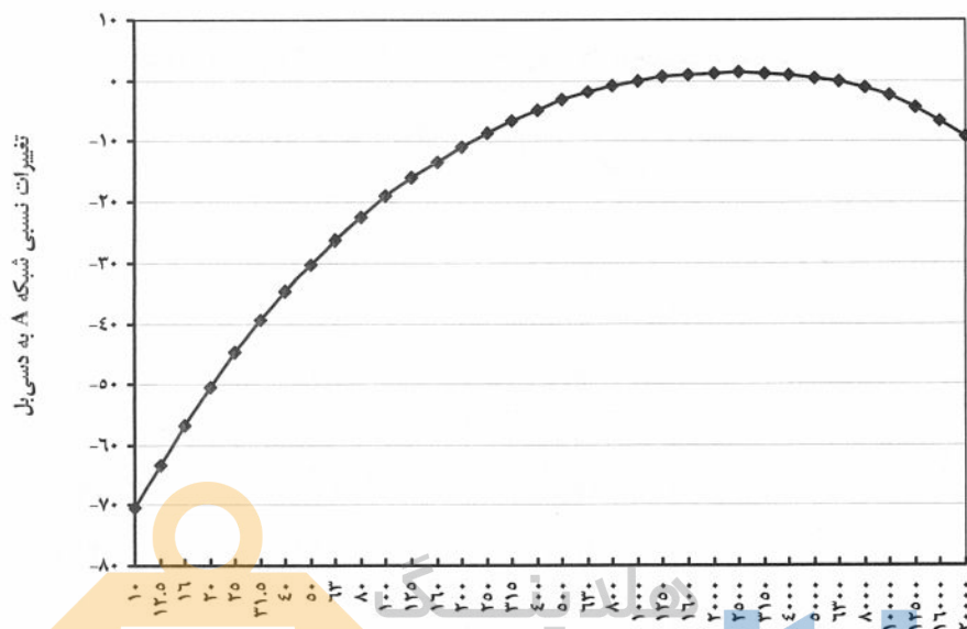
بسامد بندهای یک سوم هنگامی به هرتز شکل ۱۸-۳-۱: نمودار تغییرات نسبی شبکه وزنی A در بسامدهای مختلف
