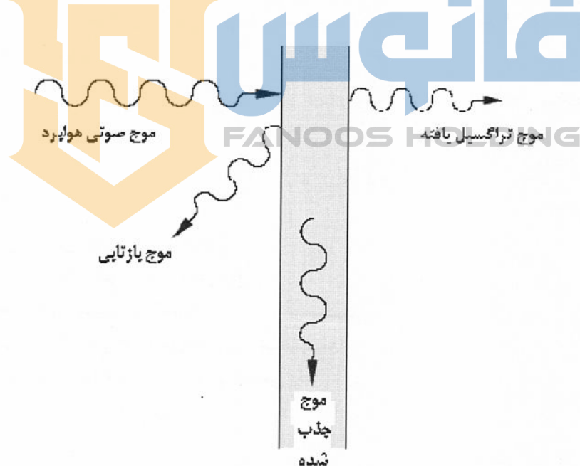
شکل ۱-۱۸-۳-۳: تراگسیل صدای هوابرد از طریق یک جداکننده
