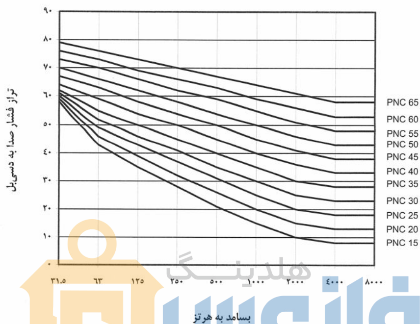
شکل ۱۸-۳-۵: نمودارهای برسنج ترجیحی نوفه PNC
