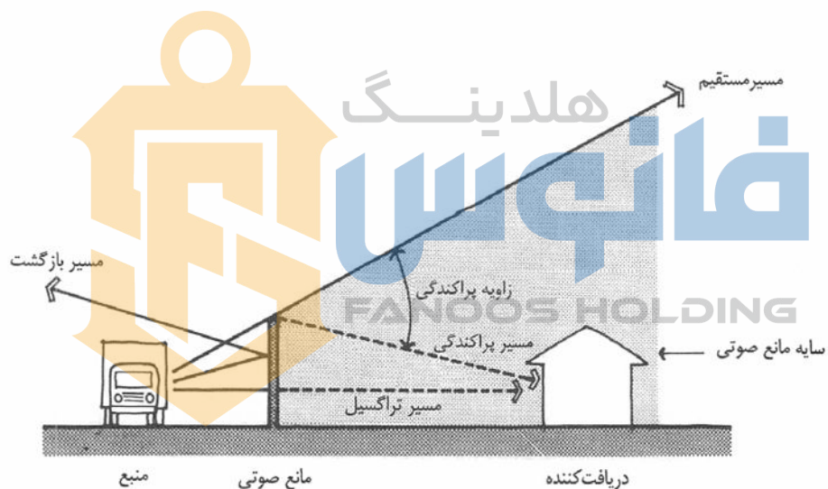
شکل پ-۴-۵: نمایش کاهش نوفه توسط مانع صوتی
