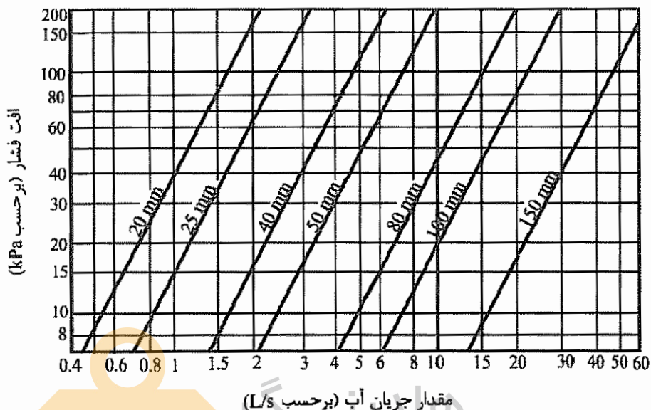
شکل پ ۴-۱ (SI) - افت فشار در کنتور نوع دیسکی بر حسب کیلوپاسکال
