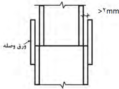
شکل ۲-۱۰-۹-۱۲ نیاز به ورق پرکننده در اتصالات جوشی
