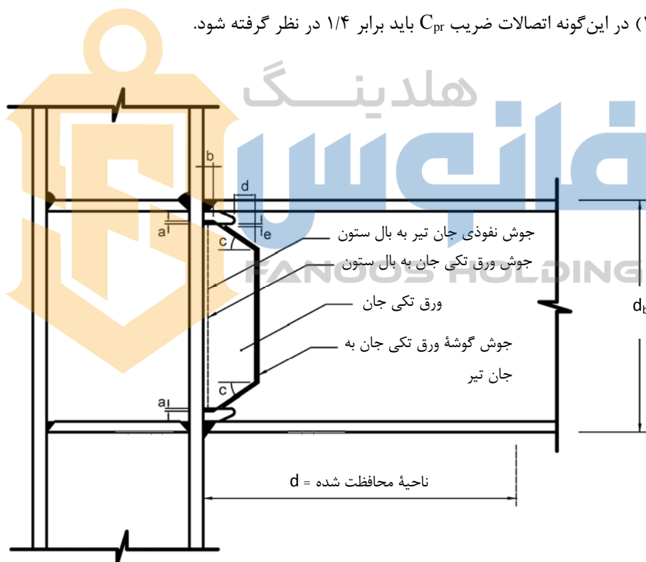
شکل ۱۰-۳-۱۳-۵ اتصال گیردار تقویت نشده جوشی (WUF-W)
