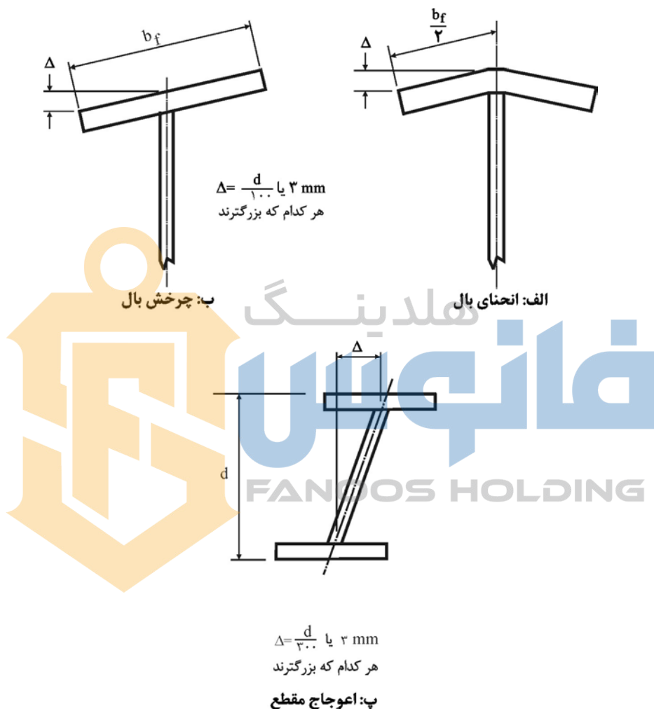
شکل ۵-۴-۱۰ رواداری‌های انحراف بال.
