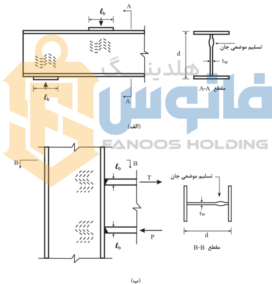
شکل ۱۰-۲-۹-۱۷ تسلیم موضعی جان در مقابل نیروی متمرکز کششی و فشاری
