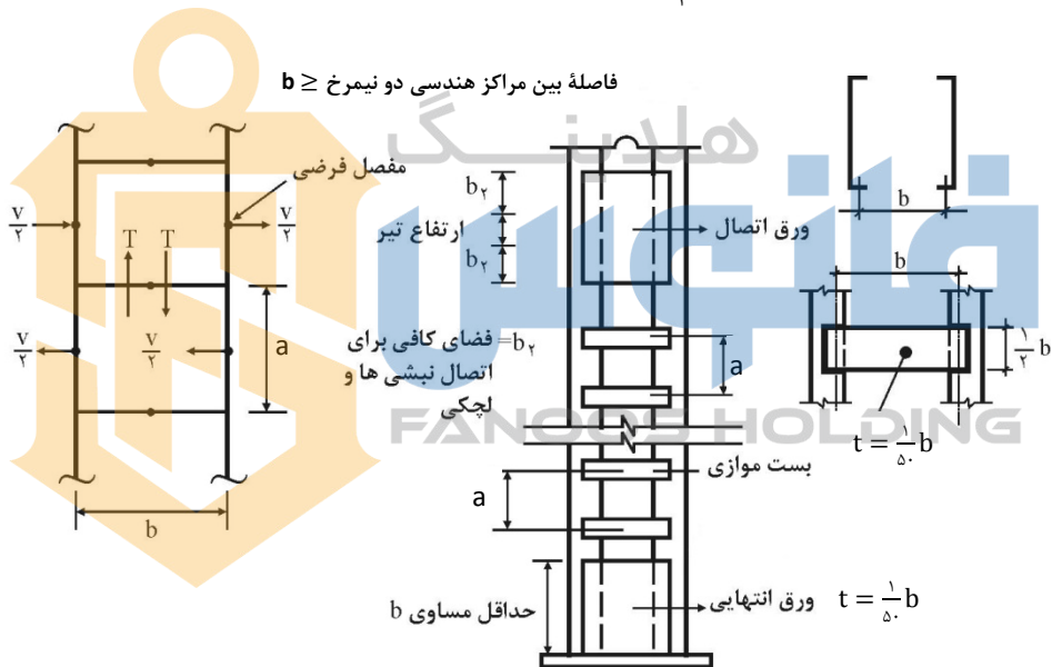
شکل ۲-۱۰-۴-۴ عضو فشاری ساخته شده با بست‌های موازی
