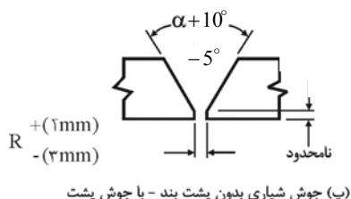
شکل ۱۰-۴-۱ رواداری‌های مونتاژ در درزها با جوش شیاری
