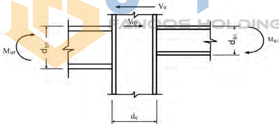
شکل ۱۰-۲-۹-۲۱ برش در چشمه اتصال
