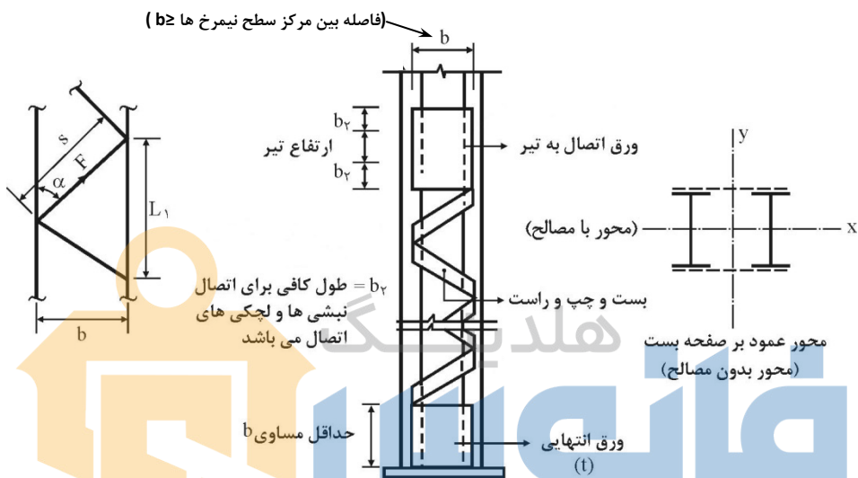
شکل ۱۰-۲-۳-۴-۵ عضو فشاری ساخته شده با بست‌های مورب
