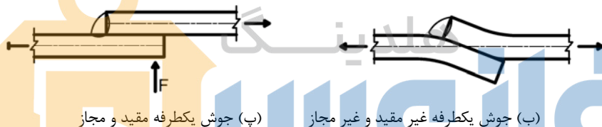
شکل ۱۰-۲-۹-۵ اتصال پوششی (رویهم) دو قطعه
