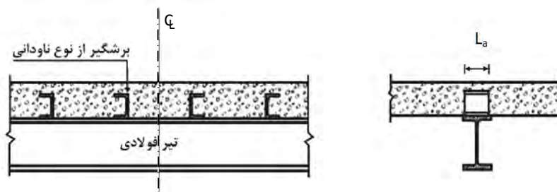
شکل ۱۰-۲-۷ برشگیرهای از نوع ناودانی
