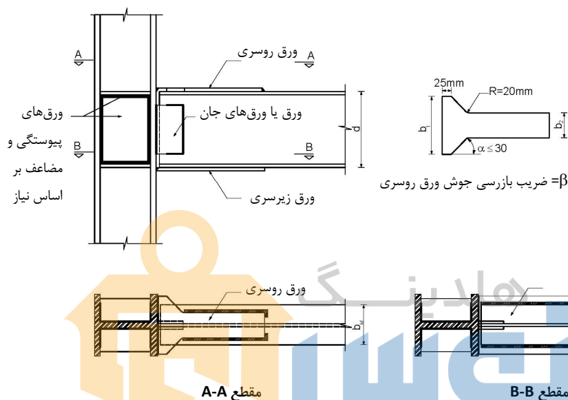
شکل ۱۰-۳-۴ اتصال گیردار جوشی به کمک ورق‌های روسری و زیرسری (WFP)
